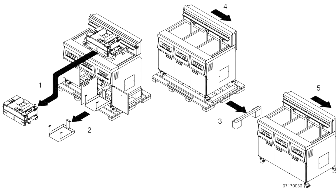
Figure 2-1 Указания по распаковке
